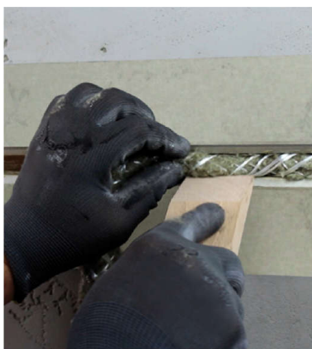
Vložte povrazec Nullifire FJ203 do špáry.
