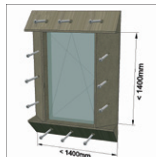
Obr. 5: Zabezpečovacie šróby 1 fig. pre špáru 10 mm
